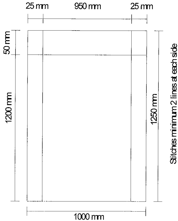
Fig : Geo-Bag (250 kg)
